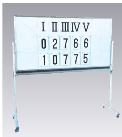
BT395 テニス用得点板 1台 ¥283,000(税別) ●キャスター付 ●巾≒1.9m×奥行≒0.55m×高さ≒1.8m 重量≒37kg
